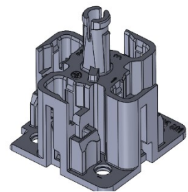
【変更後 端子台外観】
