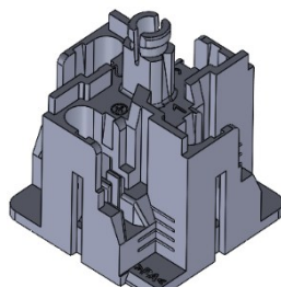
【変更前 端子台外観】
