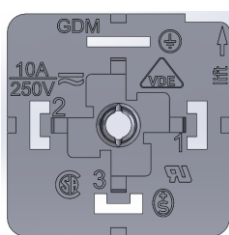
【変更前 端子台外観】
